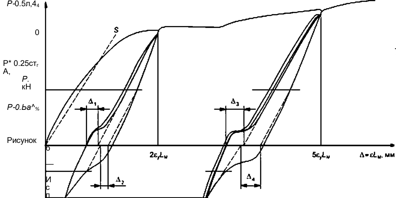
ытание при переменном растяжении и сжатии при высоком уровне пластических деформаций в механических соединениях
