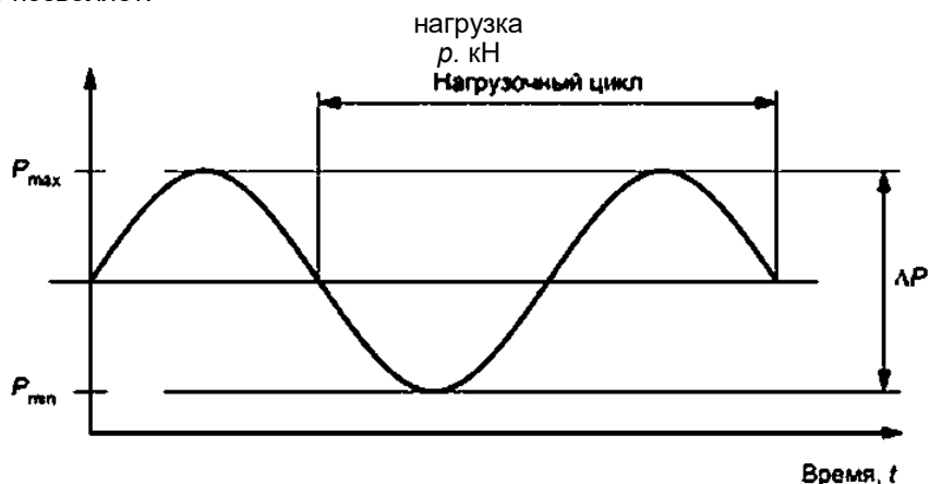
Рисунок 4 — Характеристика цикла нагрузки при испытаниях на выносливость
