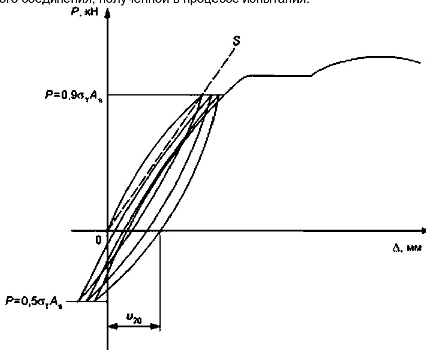
Рисунок 5 — Испытание при переменном растяжении и сжатии при высоком уровне напряжений а механических соединениях
